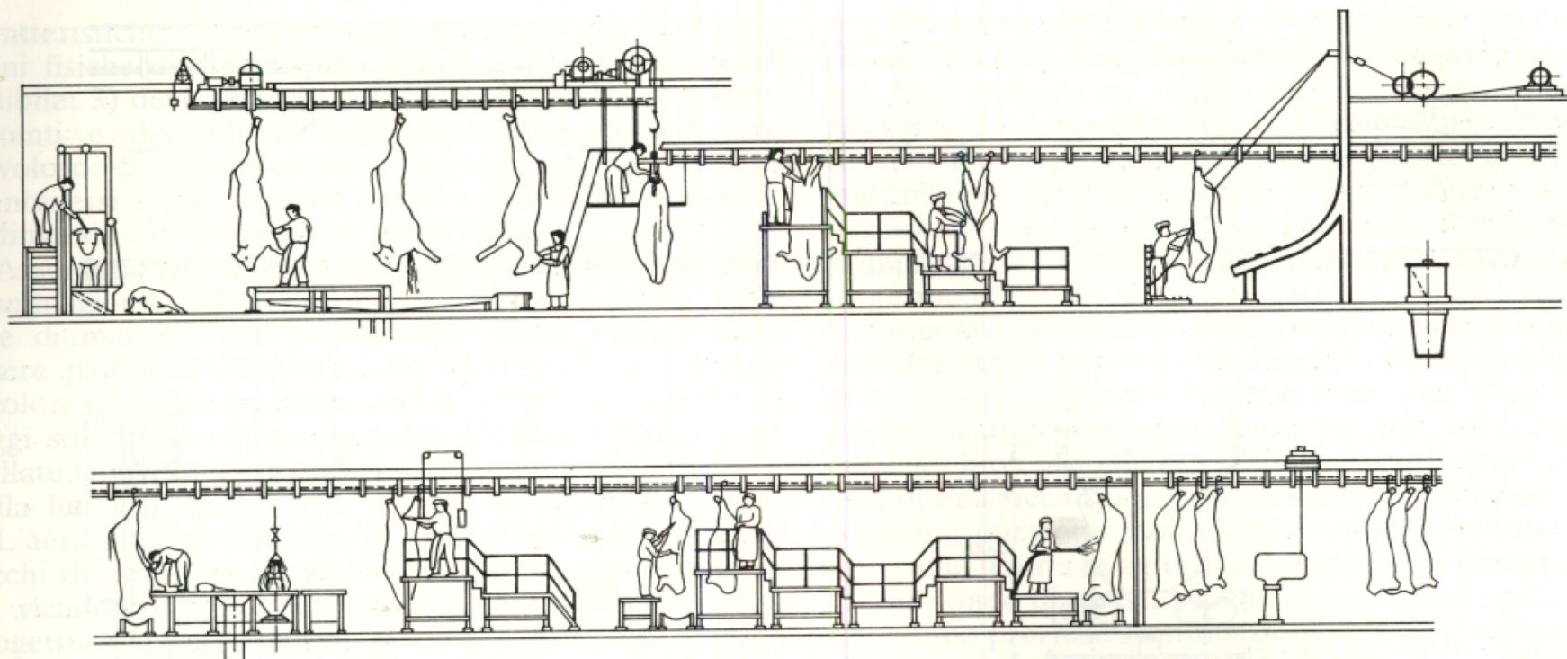
Fig. 2.2. — Catena di macellazione in sospensione per bovini. Sono sottolineate la trappola di stordimento, il dissanguamento per sgocciolamento, lo scuoimento a strappo e le varie fasi di toelettatura fino al lavaggio e pesatura delle mezzene.
