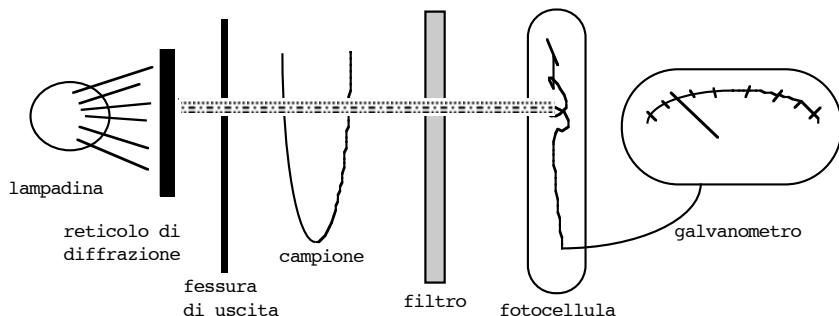
Rappresentazione schematica dello spettrofotometro impiegato per determinare la torbidità di una sospensione batterica. La luce bianca emessa da un filamento di tungsteno, colpendo un reticolo di diffrazione produce uno spettro di fotoni di differente lunghezza d'onda. Solo quei fotoni che passano attraverso la fessura di uscita raggiungono il campione (modificando la fessura di uscita si può selezionare la lunghezza d'onda desiderata). I fotoni che passano attraverso il campione vanno a eccitare una fotocellula che è collegata a un galvanometro il quale misura l'intensità luminosa. Quanto minore è la concentrazione cellulare del campione tanto maggiore è la quantità di luce emessa e viceversa. (da Boyd, Microbiologia generale, Medical Books).
