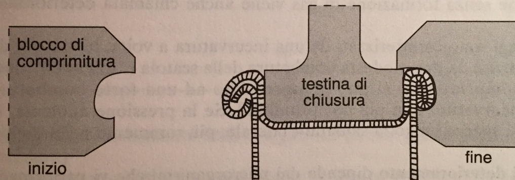
Fig. 47 - Procedimento di aggraffatura delle scatole di latta per conserve.
