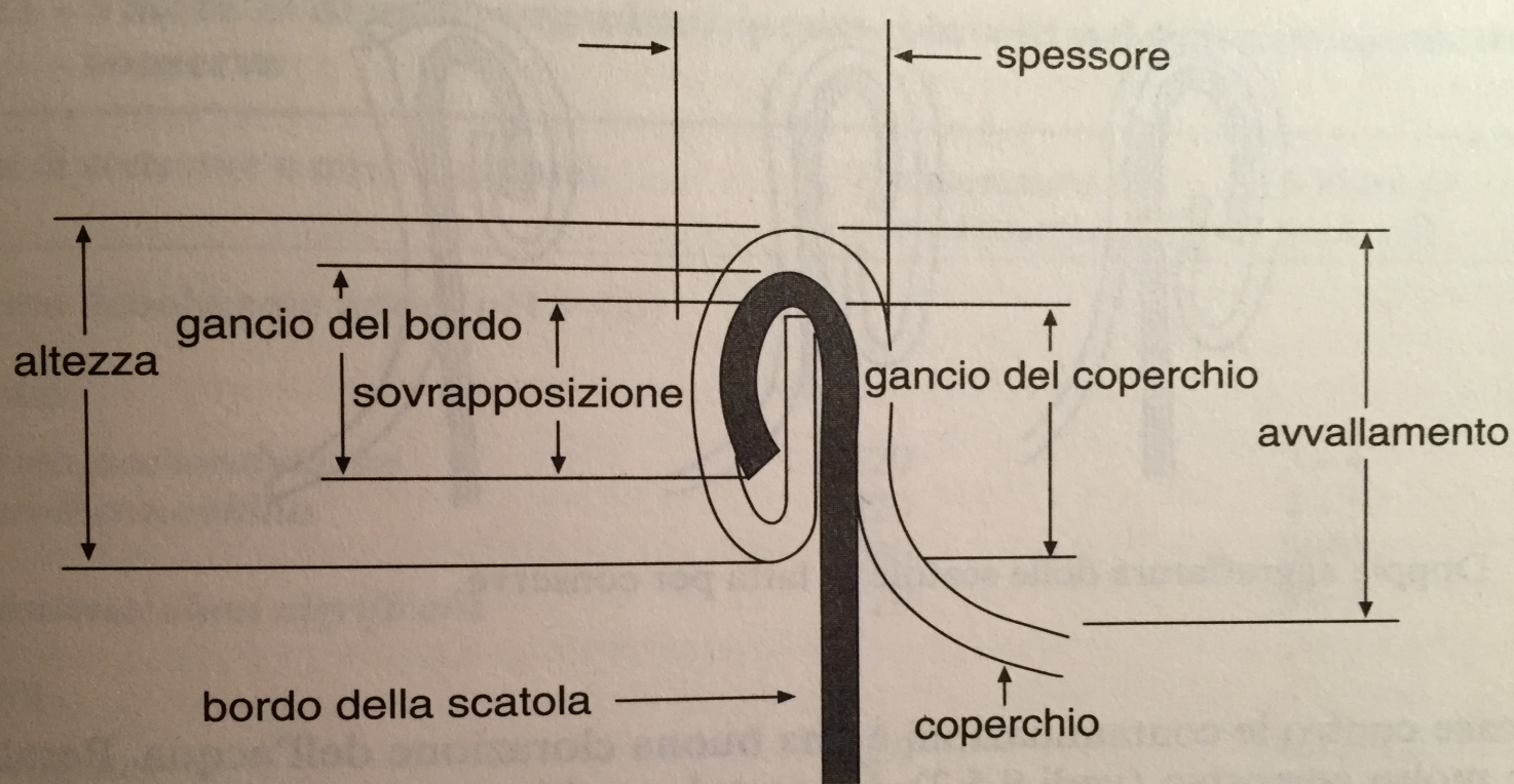
Fig. 46 - Doppia aggraffatura delle scatole di latta per conserve.
